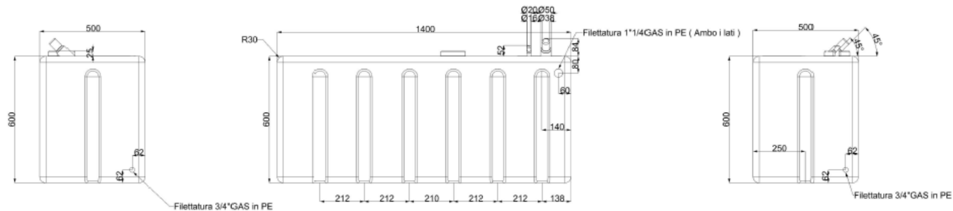
SEZ A - A
